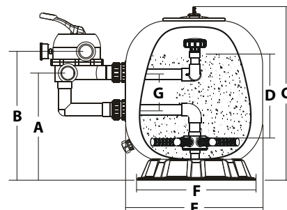
Medidas modelo: 400SA
